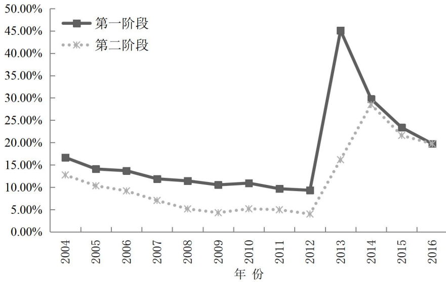
图 4 空气质量轻度污染的天数占总监测天数比例
