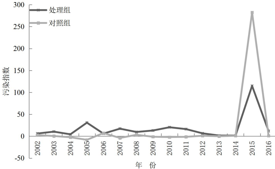
图 5 共同趋势检验
