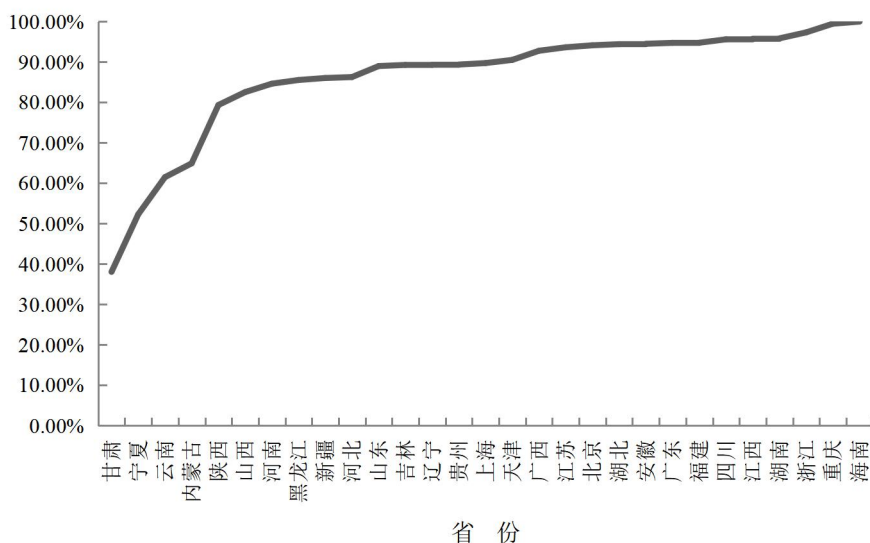
图 2 PM 2.5 、O 3 与 CO 作为首要污染物的天数占污染总天数比重
