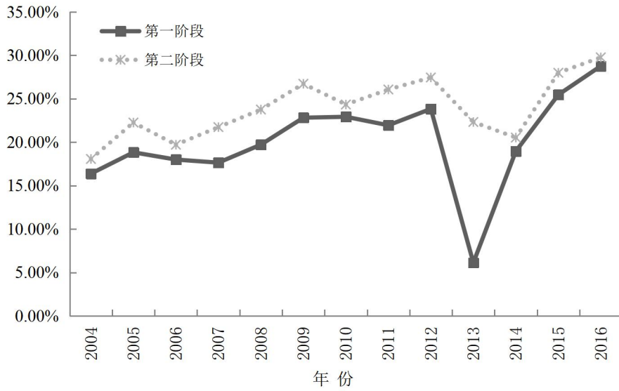
图 3 空气质量优的天数占总监测天数比例
